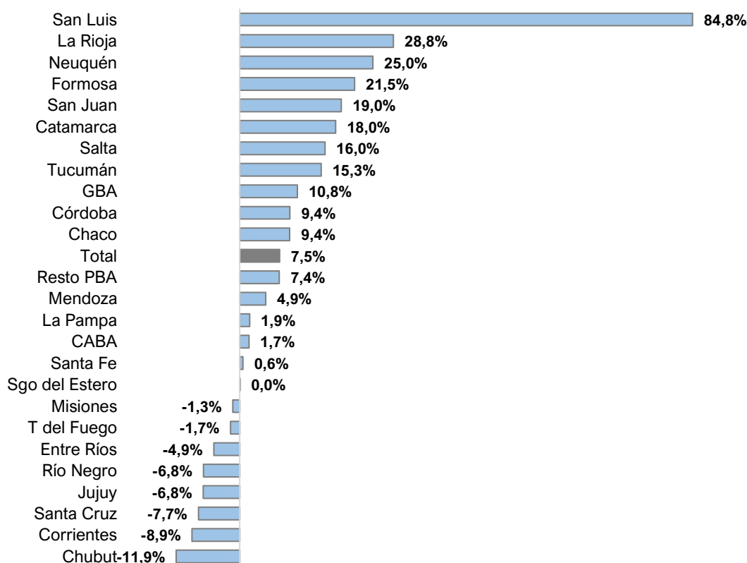
Gráfico 3. Variación % interanual. Marzo 2022. Total 25 jurisdicciones (provincia de Buenos Aires se desagrega en GBA y resto de PBA)
