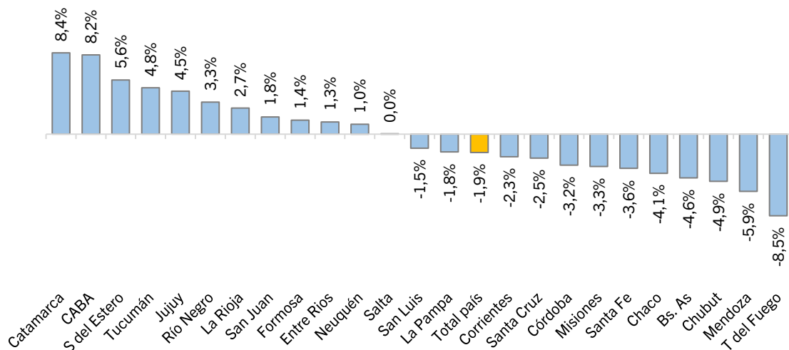
Gráfico 2. Variaciones % interanual de ventas de combustibles. Septiembre 2023. 24 jurisdicciones
